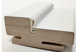
Коробка телескопич.
