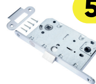
Замок и защелка BORDER ROOM, матовый хром
